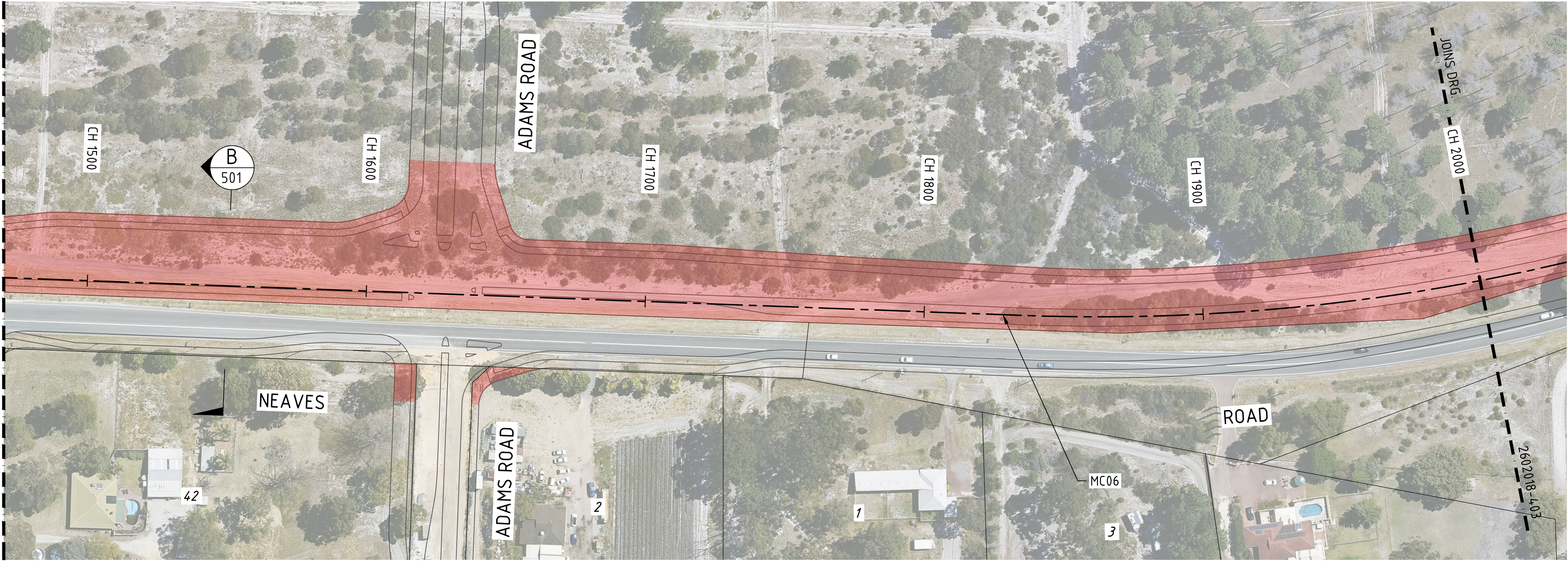
PLAN (CONT.) 1:1000
